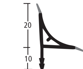
échelle 1:1 / mesure : mm
